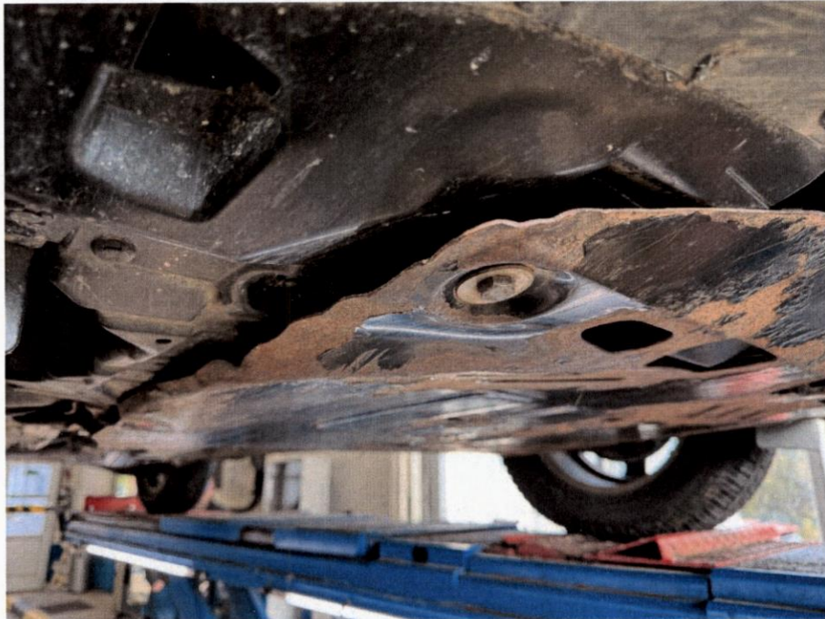
Bild 9: Unterschutz Motor verformt
